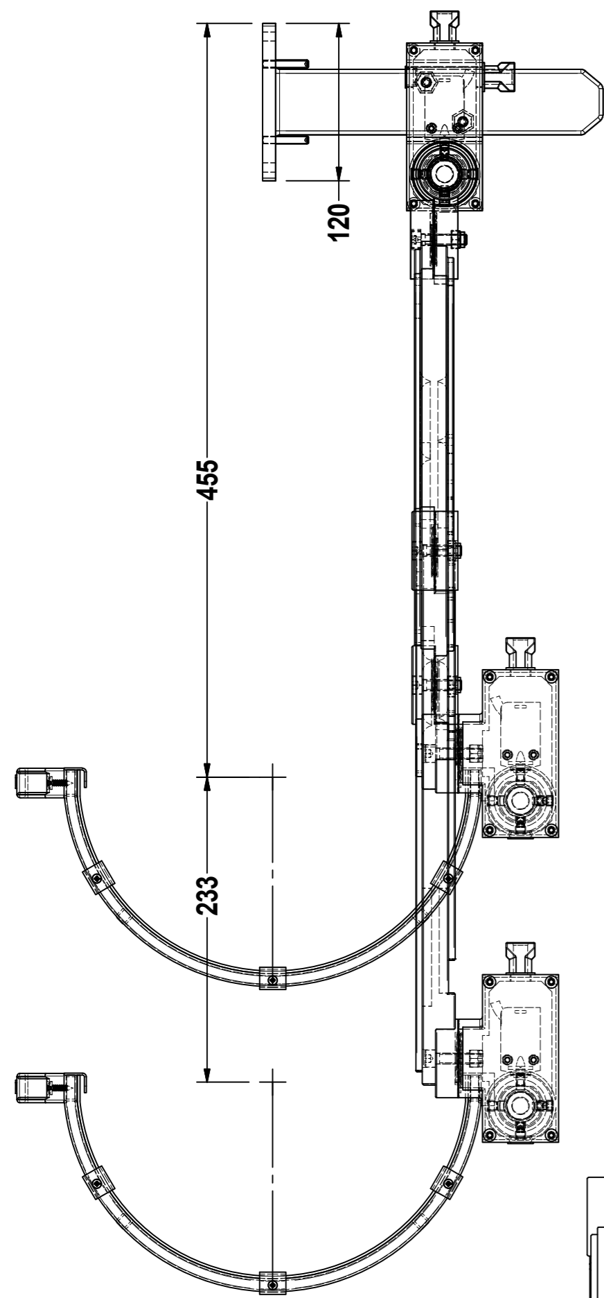
SOVRAPPOSIZIONE BRACCIO CHIUSO E BRACCIO TUTTO APERTO
